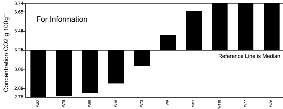
GeoPT40 - Barchart for CO2
