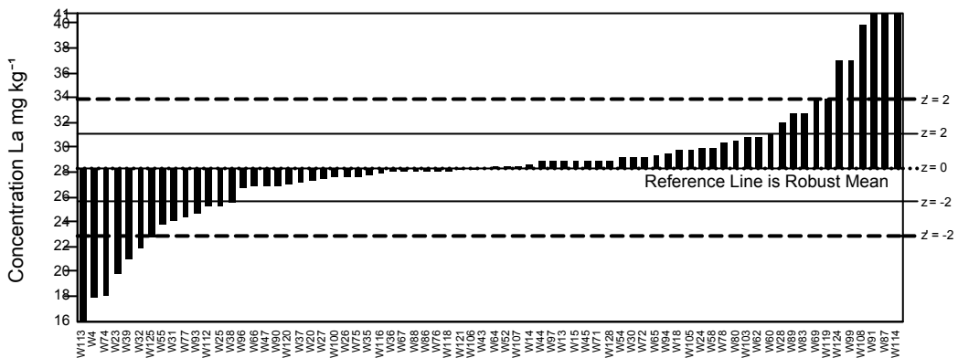
GeoPT40 - Barchart for La
