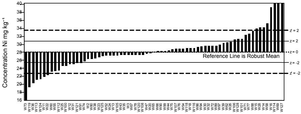
GeoPT40 - Barchart for Ni
