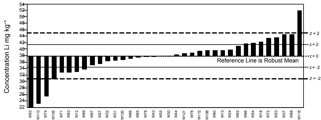
GeoPT40 - Barchart for Li
